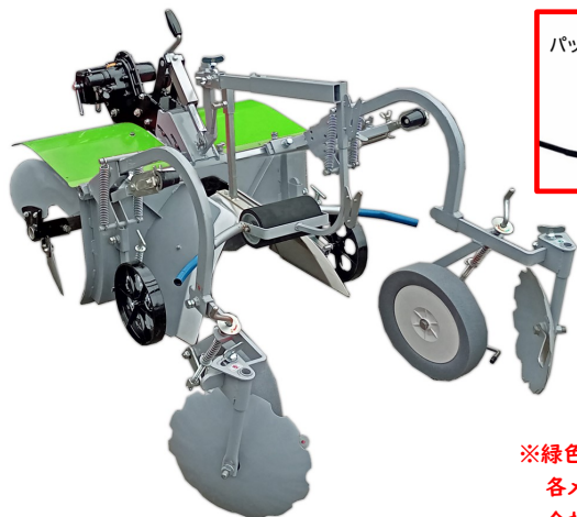
ダブル可変ベジまるこ+小うねハイマルチ
