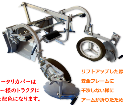
アーム折りたたみ機構・スポーク車輪 搭載
